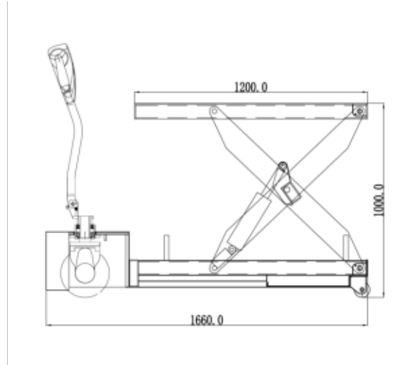
정면도 (Front)
