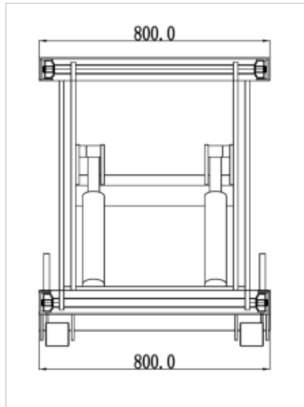
평면도 (Top)
