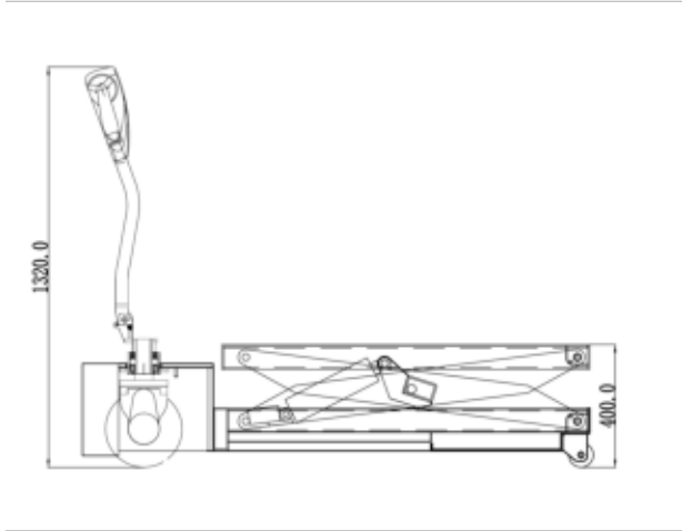
측면도 (Side)
